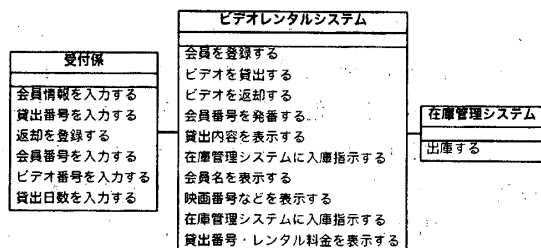
図13: ビデオレンタルシステムのクラス図
