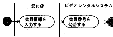
図 8: 会員を登録する
