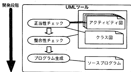
図 6: ツールの全体像
