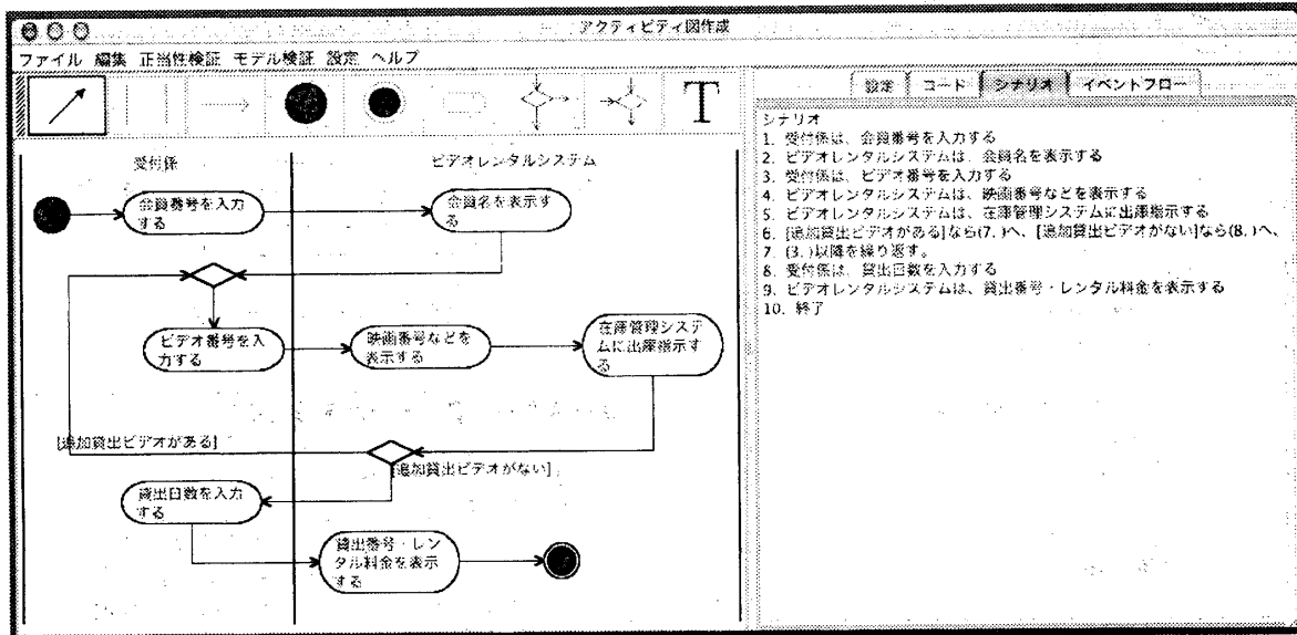
図 12: アクティビティ図作成画面
