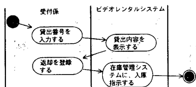
図 10: ビデオを返却する
