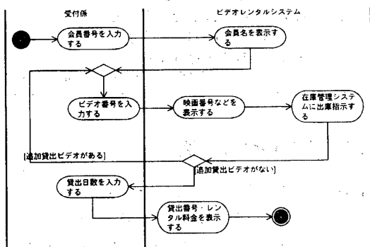
図 9: ビデオを貸出する
