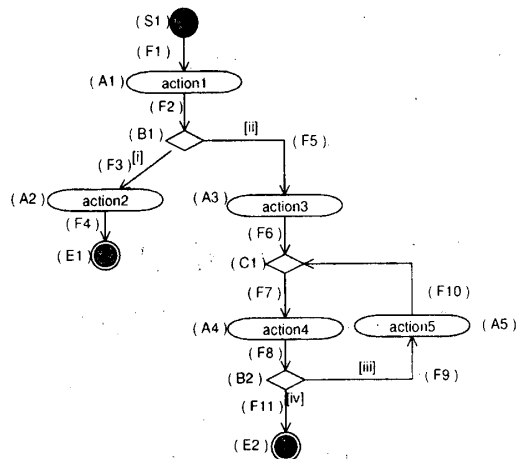
図 2: アクティビティ図の例
