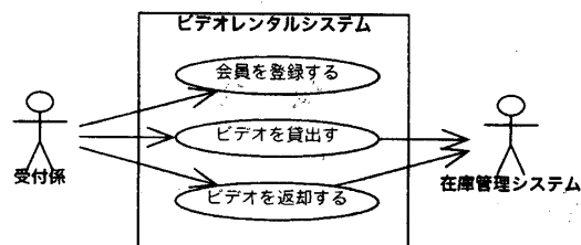
図 7: ユースケース図
