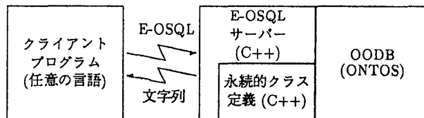
図 1: E-OSQL による OODB の利用形態
