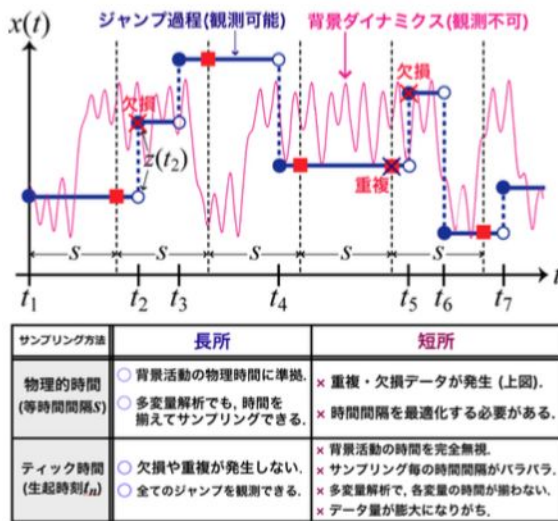
図 2: ジャンプ過程の状態値 x(t) を等時間間隔 S で観測した様子。図中の \circ が観測されるデータであり、 S の大きさに応じて欠損や重複データが発生してしまう。一方、ティック時間 t_m で観測すると、背景ダイナミクスの時間構造を破壊してしまう。
